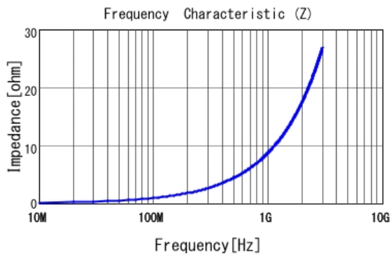
■ LQP03TN1N4BZ2 |Z|
