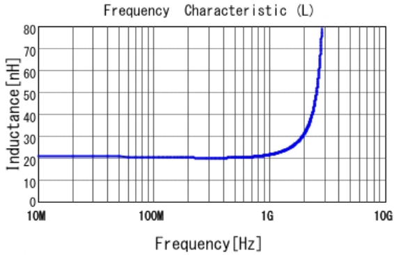
■ LQP03TN20NH02 L
