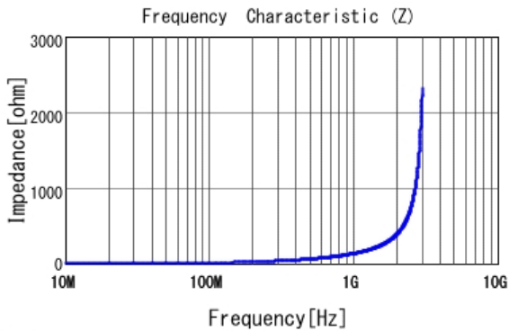
■ LQP03TN20NH02 |Z|
