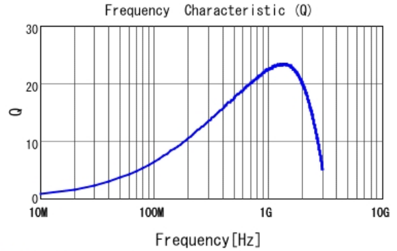
■ LQP03TN20NH02 Q
