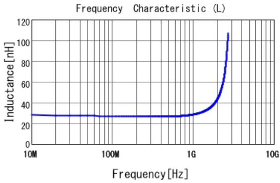
■ LQP03TN27NH02 L
