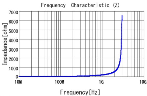
■ LQP03TN27NH02 |Z|
