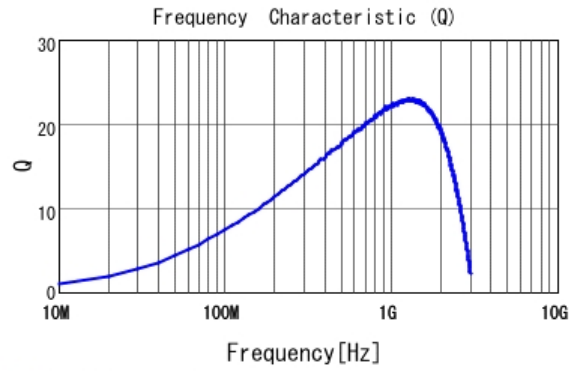
■ LQP03TN27NH02 Q
