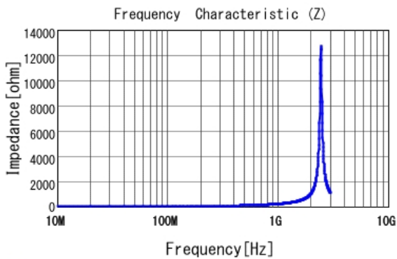
■ LQP03TN30NH02 |Z|
