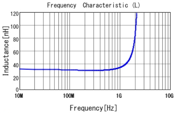
■ LQP03TN30NH02 L
