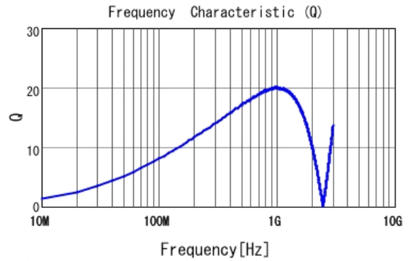
■ LQP03TN30NH02 Q
