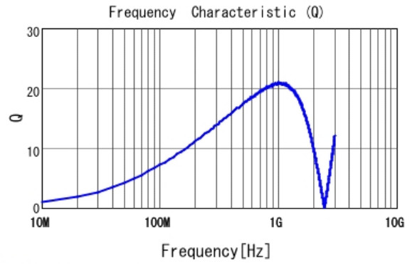
■ LQP03TN33NH02 Q
