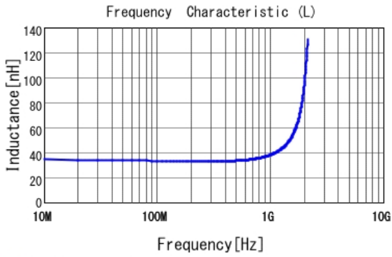
■ LQP03TN33NH02 L
