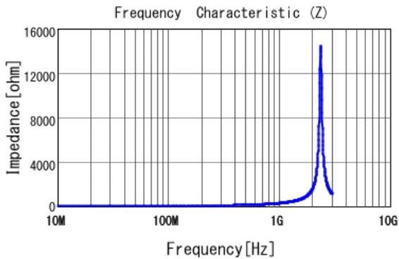
■ LQP03TN39NH02 |Z|
