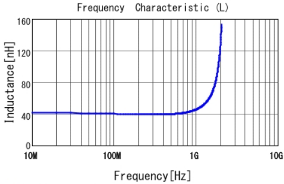
■ LQP03TN39NH02 L
