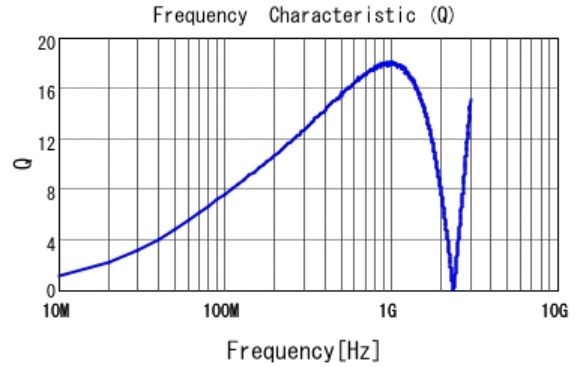
■ LQP03TN39NH02 Q
