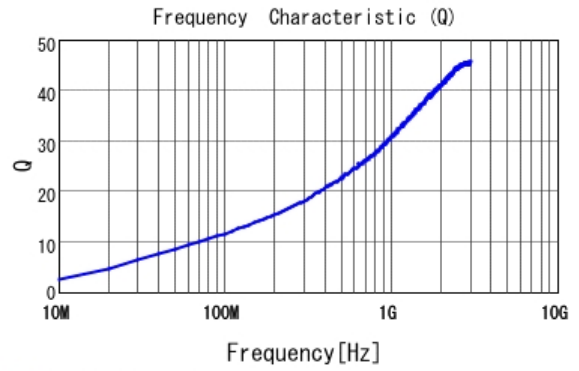
■ LQP03TN3N2B02 Q
