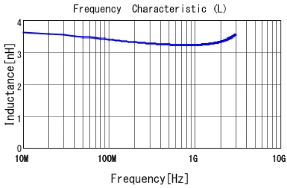
■ LQP03TN3N2B02 L
