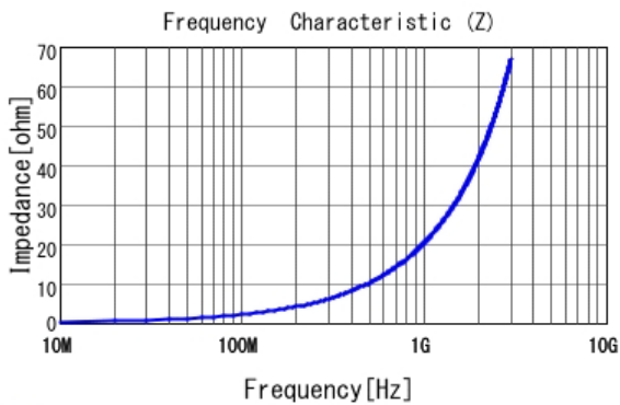
■ LQP03TN3N2B02 |Z|
