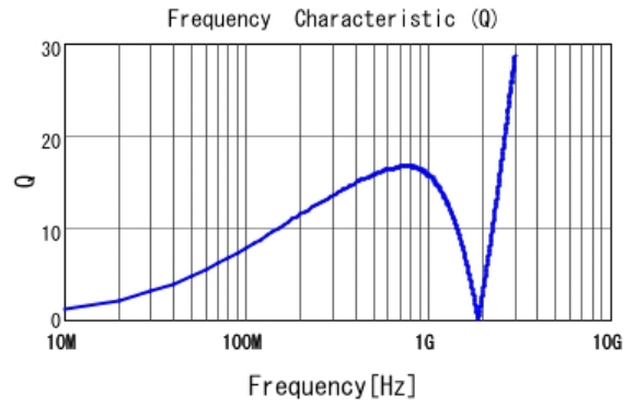
■ LQP03TN47NH02 Q
