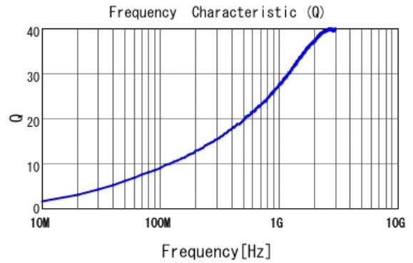
■ LQP03TN4N3H02 Q
