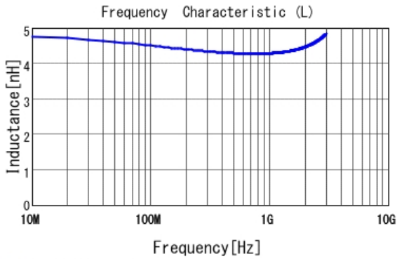
■ LQP03TN4N3H02 L
