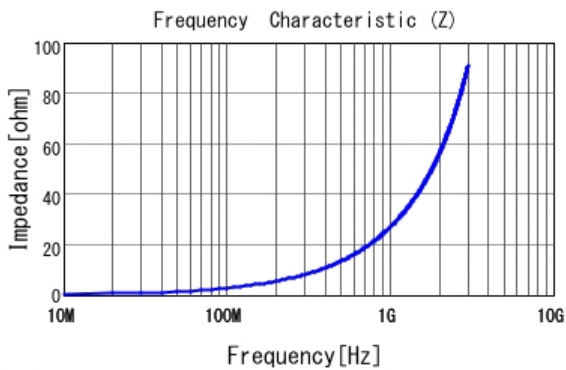
■ LQP03TN4N3H02 |Z|
