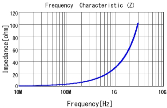
■ LQP03TN4N7H02 |Z|
