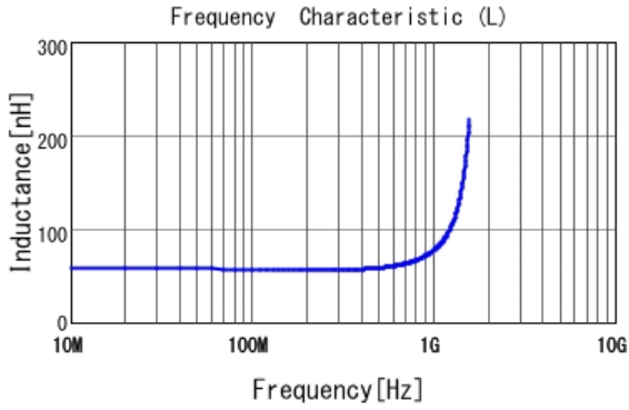
■ LQP03TN56NH02 L
