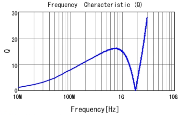
■ LQP03TN56NH02 Q
