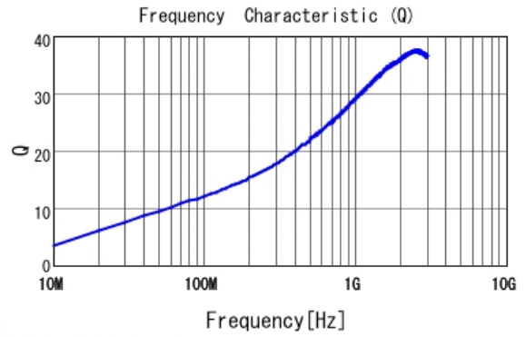
■ LQP03TN5N1H02 Q
