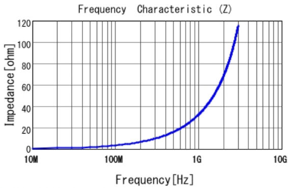
■ LQP03TN5N1H02 |Z|
