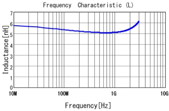
■ LQP03TN5N1H02 L
