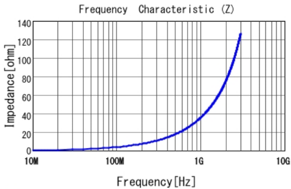
■ LQP03TN5N6H02 |Z|
