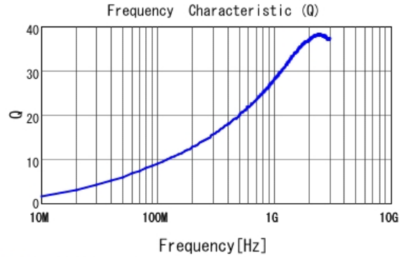
■ LQP03TN5N6H02 Q
