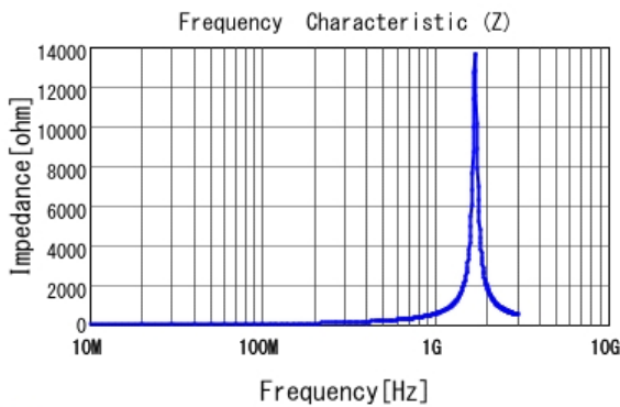
■ LQP03TN62NH02 |Z|
