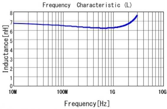
■ LQP03TN6N2H02 L
