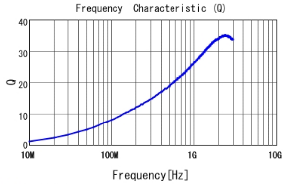
■ LQP03TN6N2H02 Q
