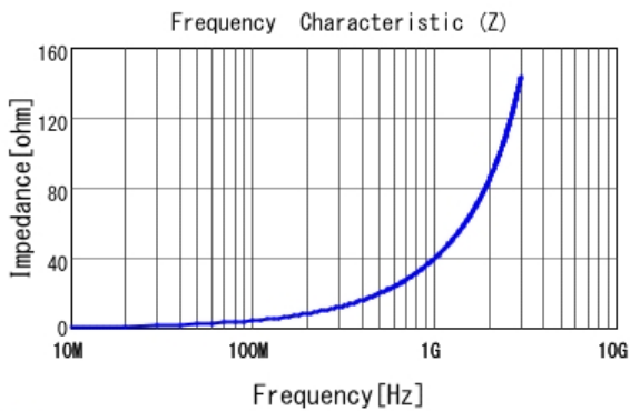
■ LQP03TN6N2H02 |Z|
