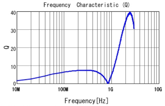
■ LQP03TNR15H02 Q
