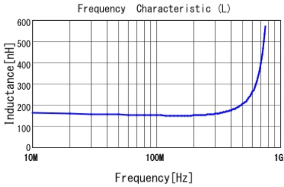
■ LQP03TNR15H02 L
