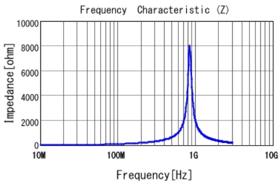
■ LQP03TNR15H02 |Z|
