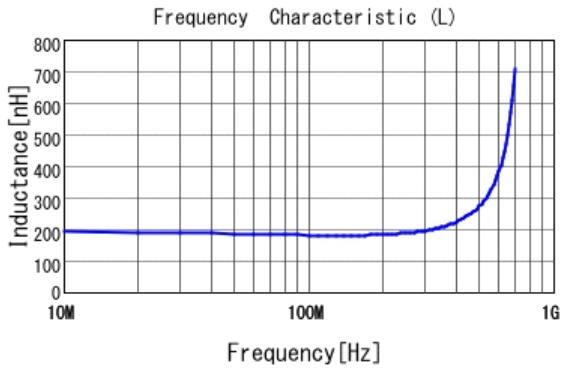
■ LQP03TNR18H02 L
