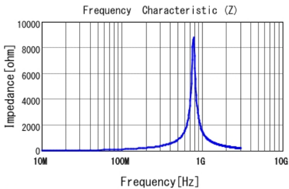
■ LQP03TNR18H02 |Z|
