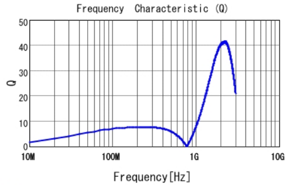
■ LQP03TNR18H02 Q
