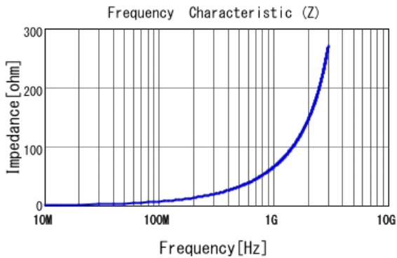
■ LQP03TQ10NH02 |Z|
