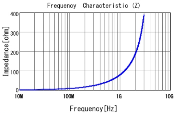
■ LQP03TQ12NJ02 |Z|
