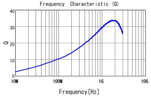
■ LQP03TQ12NJ02 Q
