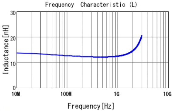
■ LQP03TQ12NJ02 L
