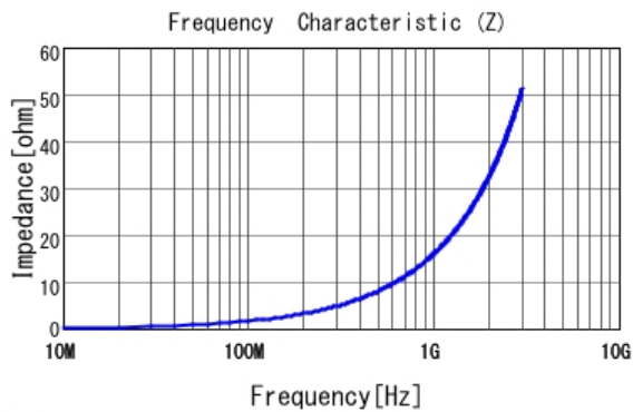
■ LQP03TQ2N5B02 |Z|
