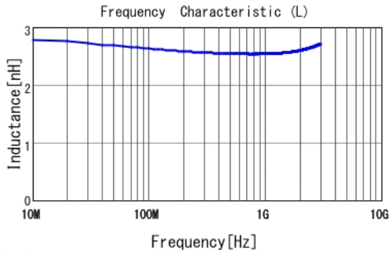
■ LQP03TQ2N5B02 L
