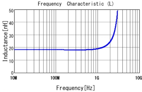
■ LQP15MN18NG02 L
