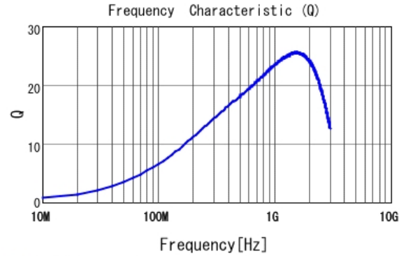
■ LQP15MN18NG02 Q
