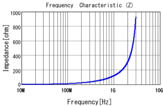
■ LQP15MN18NG02 |Z|
