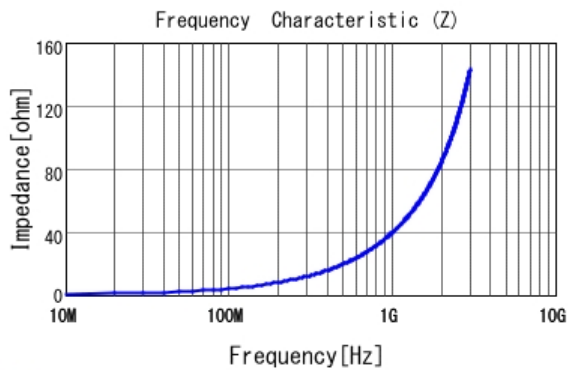
■ LQP15MN6N2B02 |Z|
