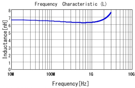
■ LQP15MN6N2B02 L
