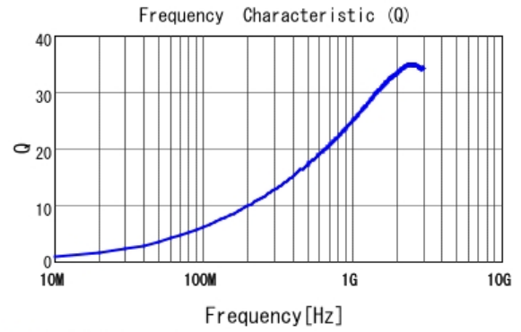
■ LQP15MN6N2B02 Q
