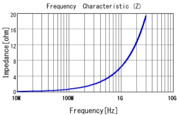
■ LQW04AN1N1D00 |Z|
