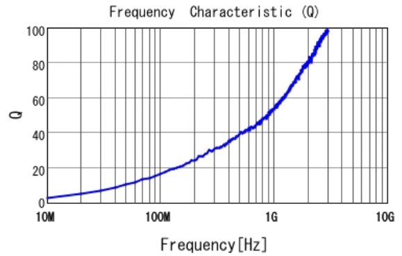
■ LQW04AN1N1D00 Q
