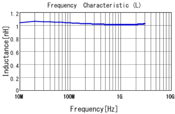
■ LQW04AN1N1D00 L
