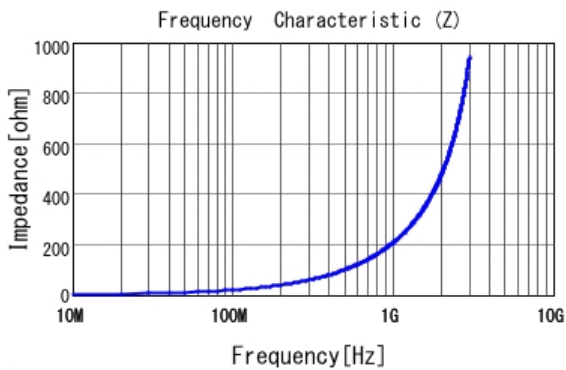
■ LQW04AN33NH00 |Z|
