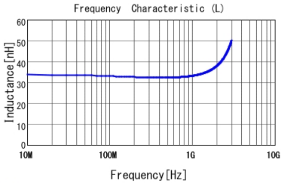
■ LQW04AN33NH00 L
