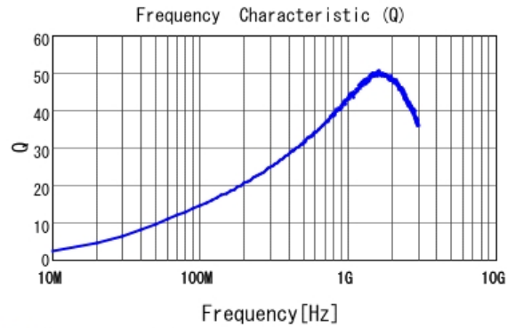
■ LQW04AN33NH00 Q
