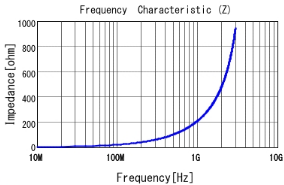
■ LQW04AN33NJ00 |Z|
