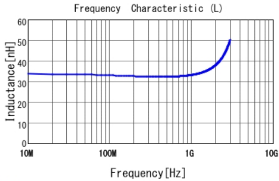
■ LQW04AN33NJ00 L
