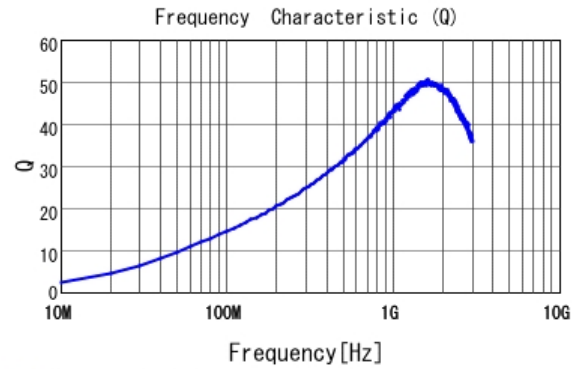
■ LQW04AN33NJ00 Q
