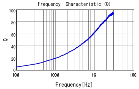
■ LQW15AN11NG00 Q
