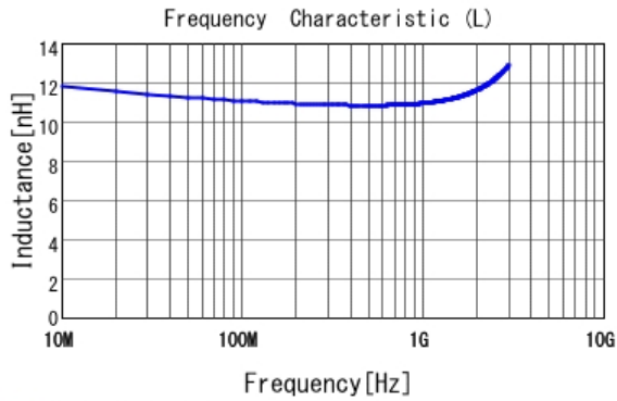
■ LQW15AN11NJ00 L
