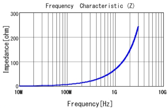
■ LQW15AN11NJ00 |Z|
