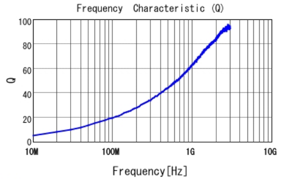
■ LQW15AN11NJ00 Q
