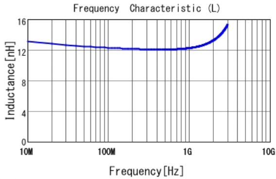
■ LQW15AN12NH00 L
