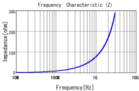
■ LQW15AN12NH00 |Z|
