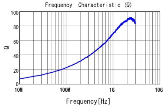
■ LQW15AN12NH00 Q
