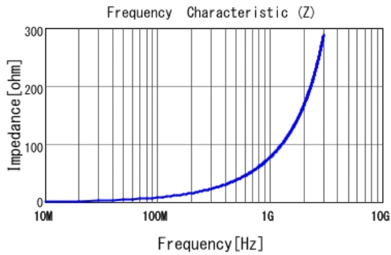
■ LQW15AN12NJ00 |Z|
