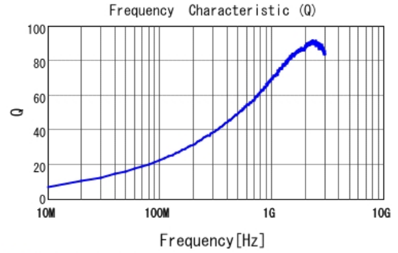
■ LQW15AN12NJ00 Q
