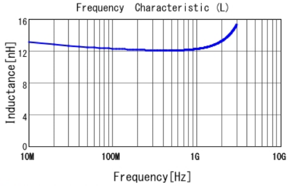
■ LQW15AN12NJ00 L
