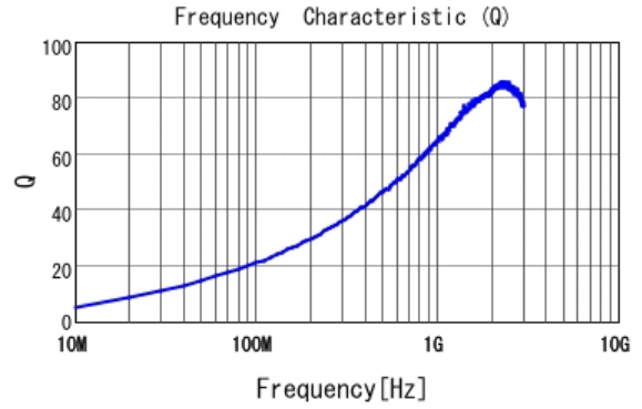
■ LQW15AN13NG00 Q
