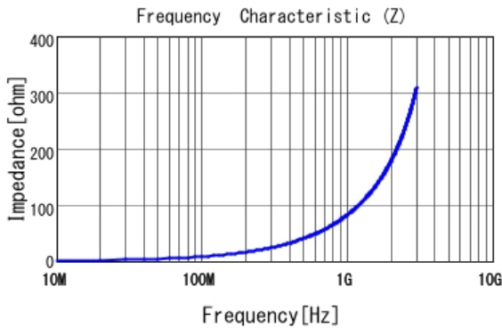
■ LQW15AN13NG00 |Z|
