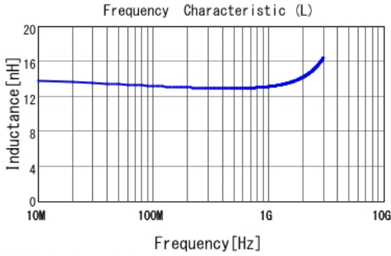
■ LQW15AN13NG00 L
