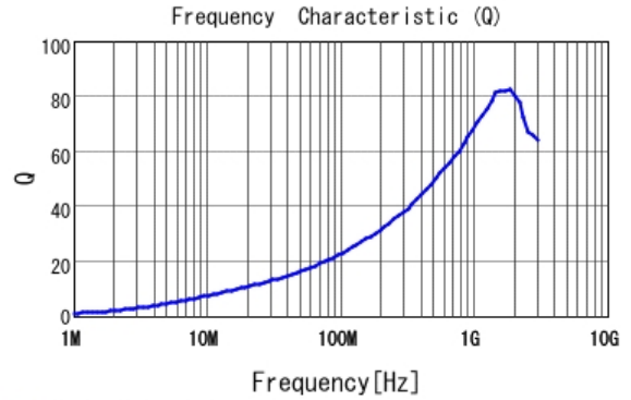
■ LQW15AN14NG80 Q
