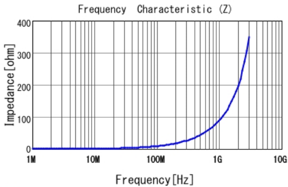
■ LQW15AN14NG80 |Z|
