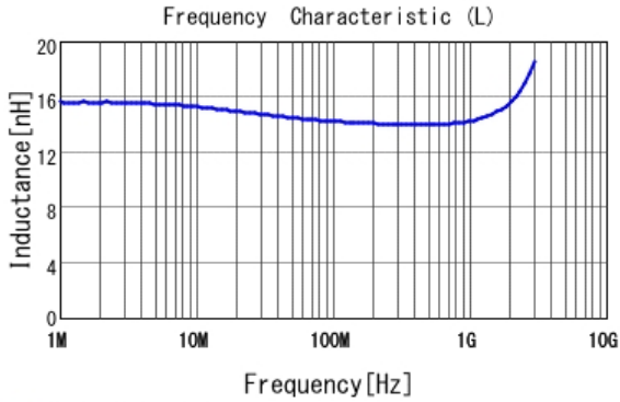
■ LQW15AN14NG80 L
