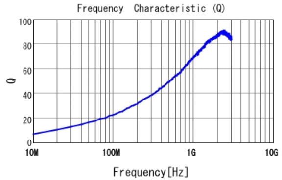
■ LQW15AN15NG00 Q
