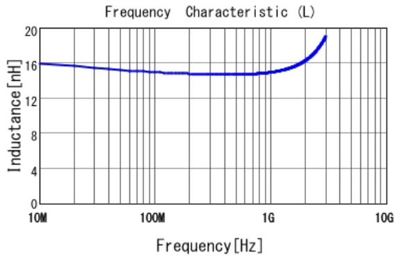
■ LQW15AN15NG00 L
