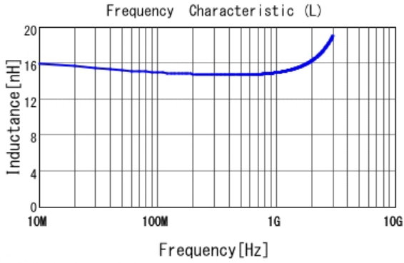
■ LQW15AN15NH00 L
