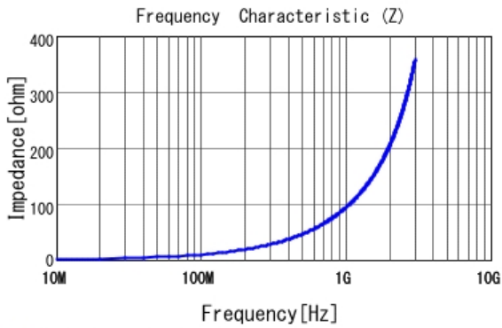
■ LQW15AN15NH00 |Z|
