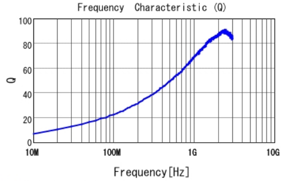
■ LQW15AN15NH00 Q
