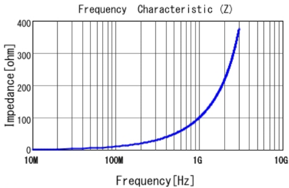
■ LQW15AN16NH00 |Z|
