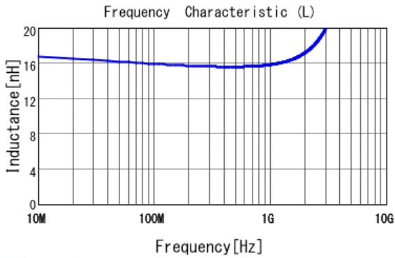
■ LQW15AN16NH00 L
