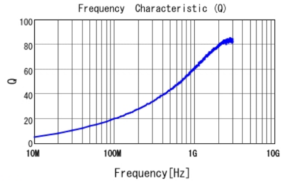
■ LQW15AN16NH00 Q
