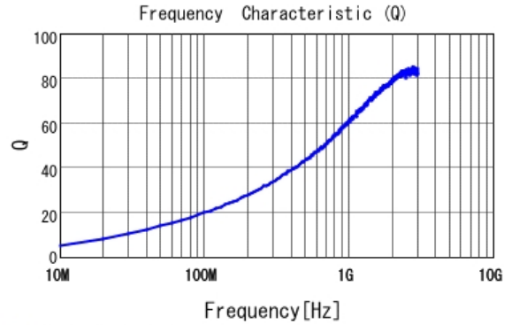
■ LQW15AN16NJ0Z Q
