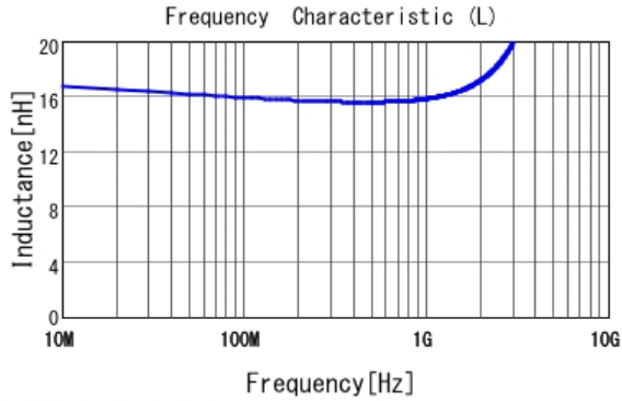
■ LQW15AN16NJ0Z L
