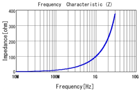
■ LQW15AN16NJ0Z |Z|
