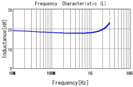
■ LQW15AN18NJ00 L
