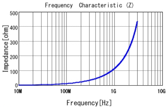
■ LQW15AN18NJ00 |Z|
