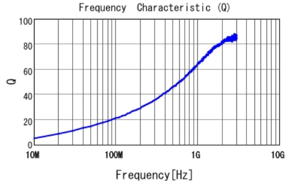
■ LQW15AN18NJ00 Q
