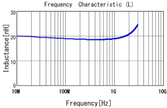
■ LQW15AN19NG00 L
