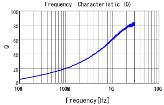
■ LQW15AN19NG00 Q
