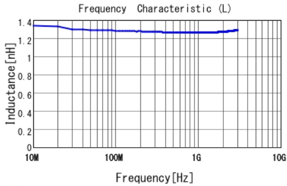
■ LQW15AN1N3C10 L
