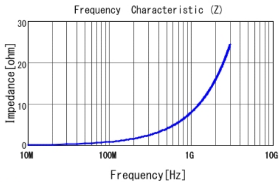
■ LQW15AN1N3C10 |Z|
