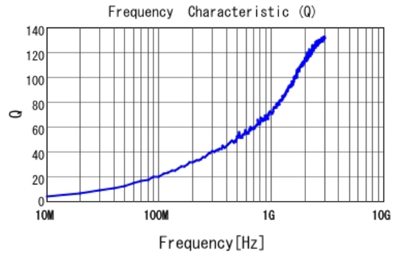
■ LQW15AN1N3C10 Q
