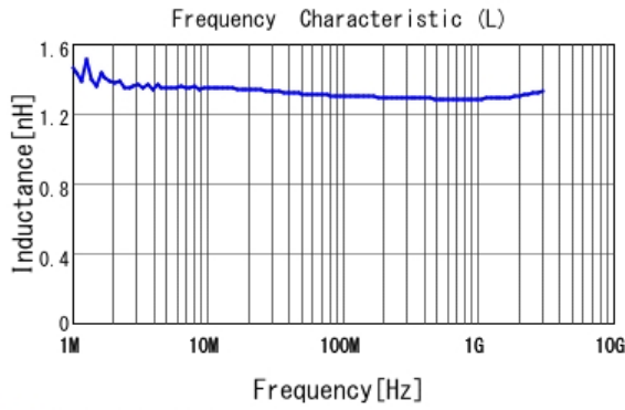
■ LQW15AN1N3C80 L
