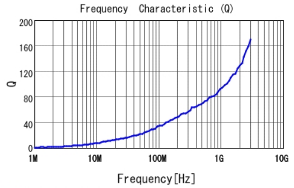
■ LQW15AN1N3C80 Q
