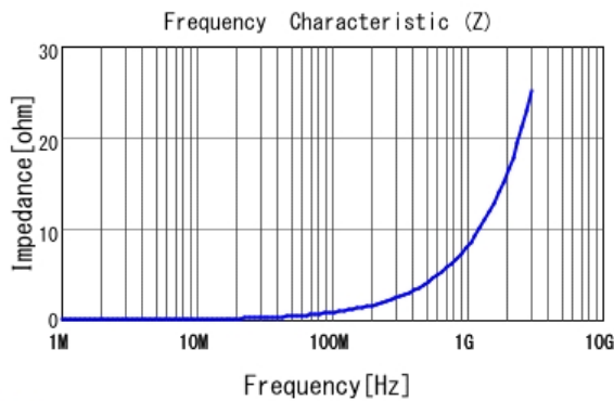
■ LQW15AN1N3C80 |Z|
