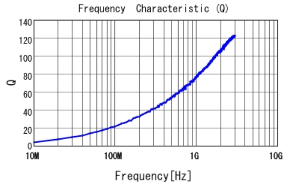
■ LQW15AN1N4C10 Q
