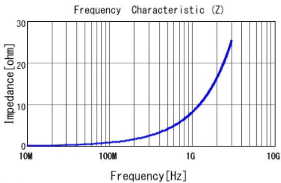
■ LQW15AN1N4C10 |Z|
