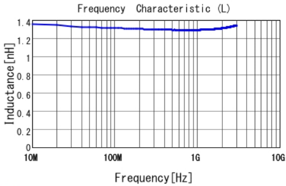
■ LQW15AN1N4C10 L
