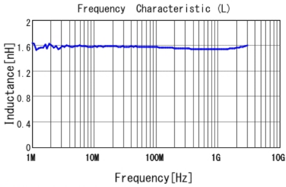
■ LQW15AN1N6C8Z L
