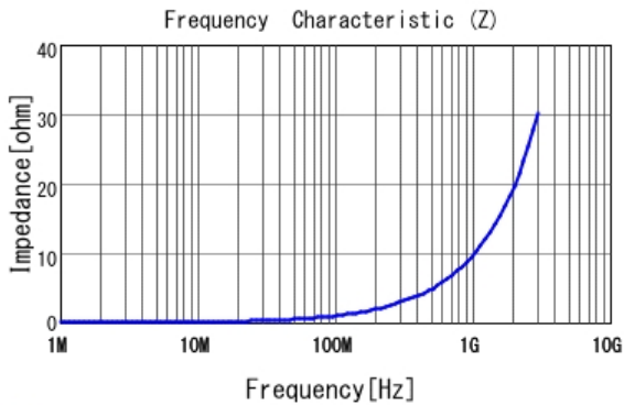
■ LQW15AN1N6C8Z |Z|
