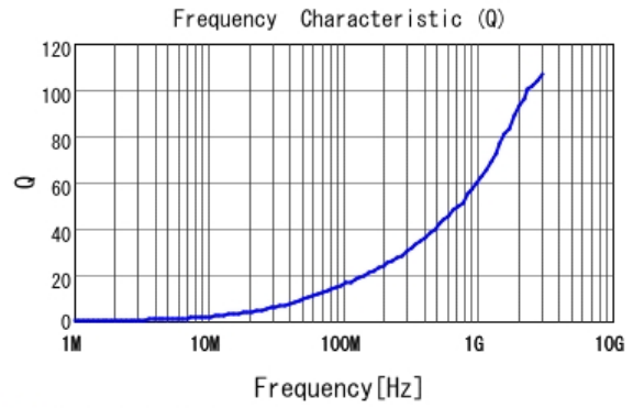
■ LQW15AN1N6C8Z Q
