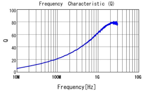
■ LQW15AN20NG00 Q
