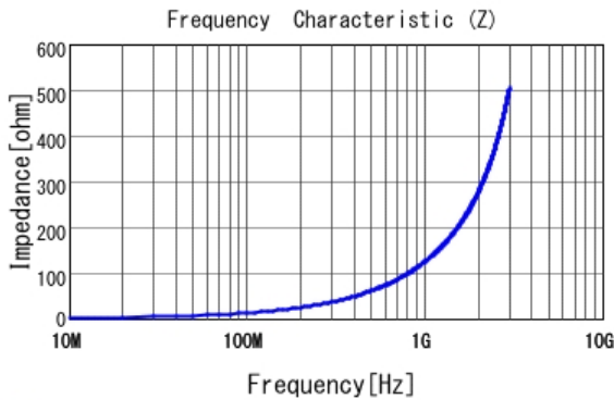
■ LQW15AN20NG00 |Z|
