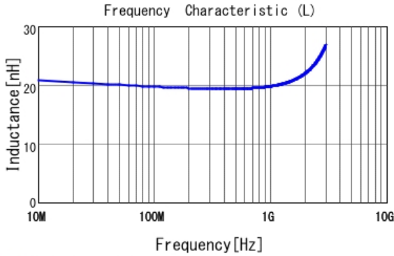
■ LQW15AN20NG00 L
