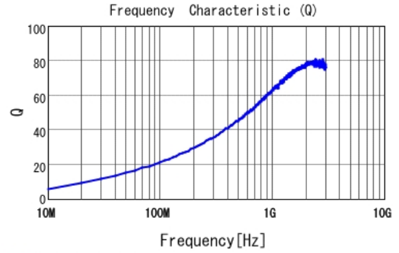
■ LQW15AN20NJ00 Q
