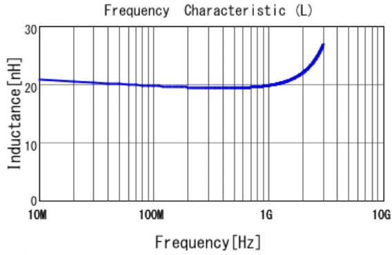
■ LQW15AN20NJ00 L
