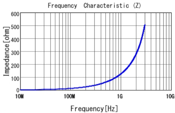
■ LQW15AN20NJ00 |Z|
