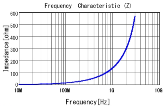
■ LQW15AN22NJ00 |Z|
