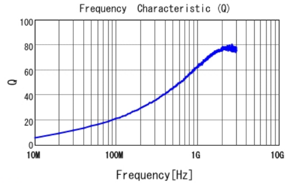
■ LQW15AN22NJ00 Q
