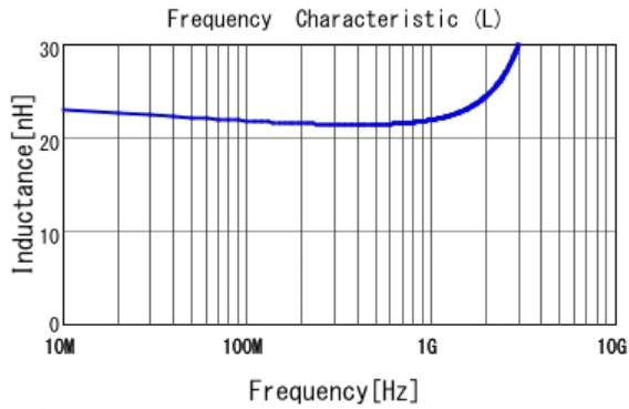
■ LQW15AN22NJ00 L
