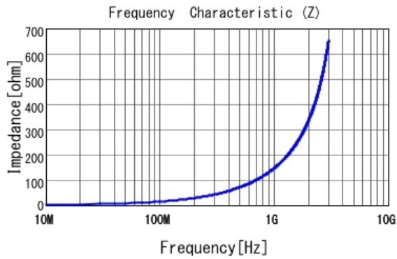
■ LQW15AN23NG00 |Z|
