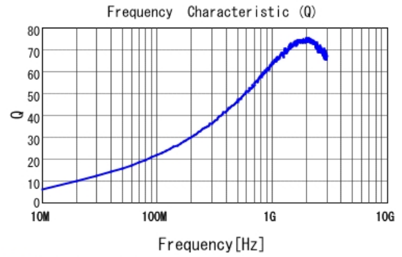
■ LQW15AN23NG00 Q
