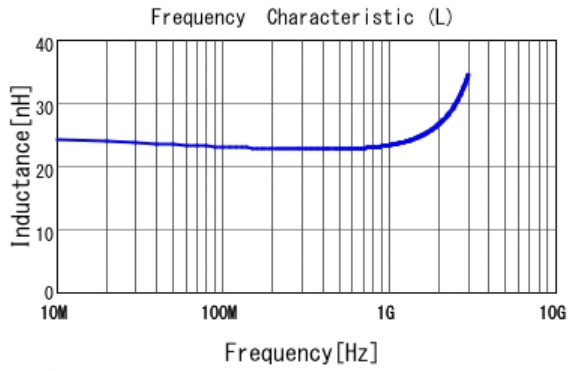
■ LQW15AN23NG00 L
