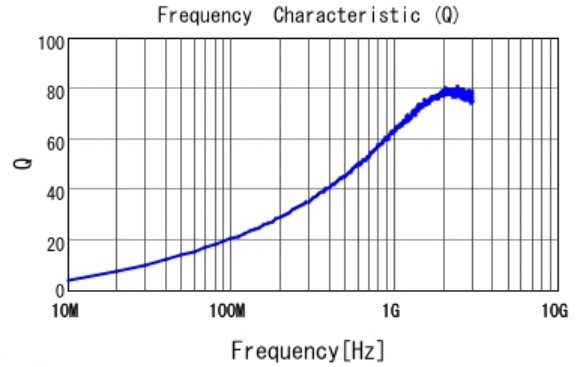
■ LQW15AN24NG00 Q
