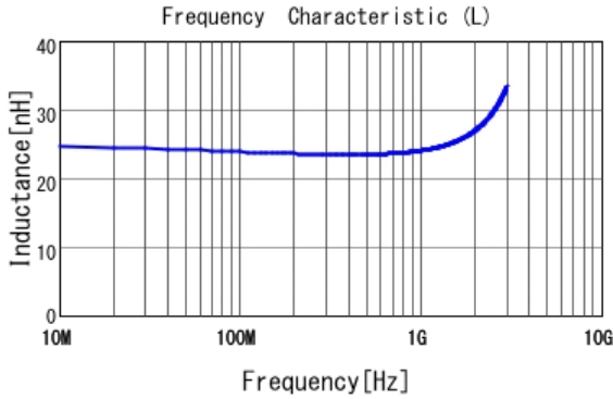
■ LQW15AN24NG00 L
