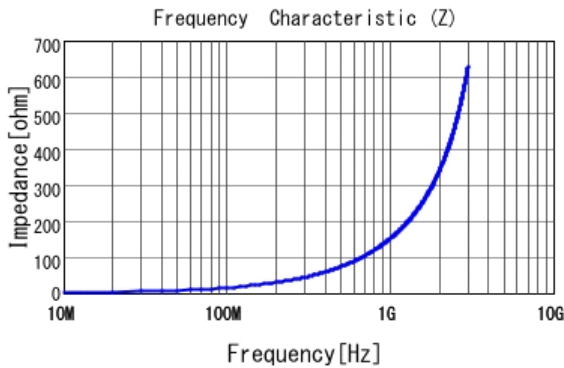
■ LQW15AN24NG00 |Z|
