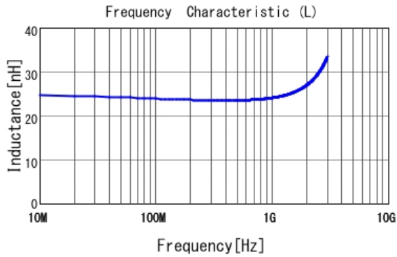
■ LQW15AN24NJ00 L
