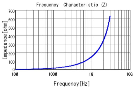
■ LQW15AN24NJ00 |Z|
