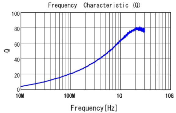
■ LQW15AN24NJ00 Q
