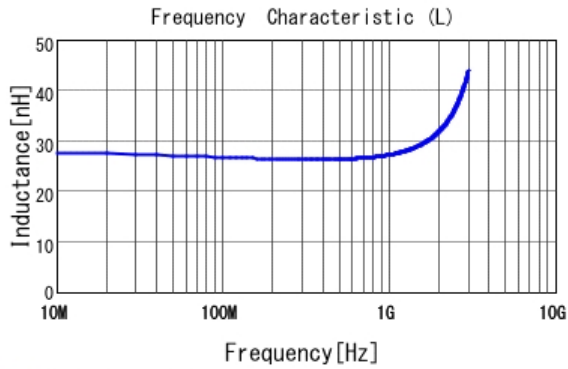
■ LQW15AN27NG00 L
