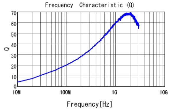
■ LQW15AN27NG00 Q
