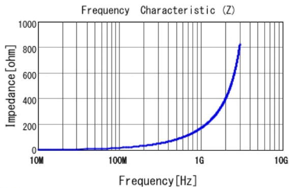
■ LQW15AN27NG00 |Z|
