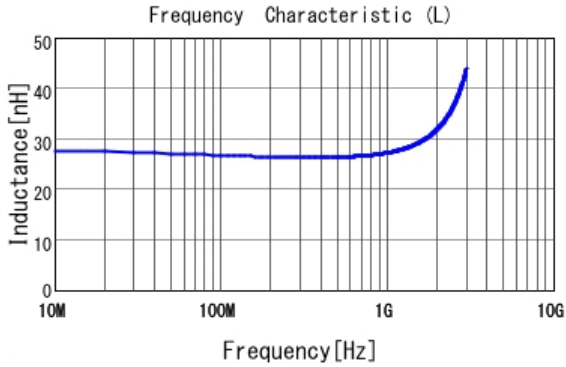
■ LQW15AN27NH00 L
