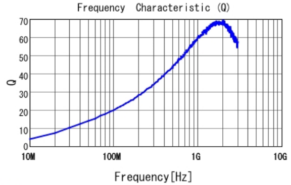
■ LQW15AN27NH00 Q
