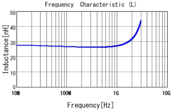
■ LQW15AN27NJ00 L
