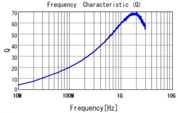
■ LQW15AN27NJ00 Q
