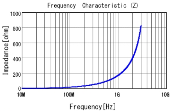
■ LQW15AN27NJ00 |Z|
